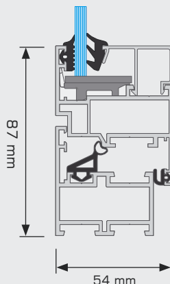
przekrój okna
