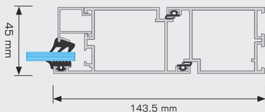
przekrój drzwi
