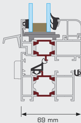
przekrój okna
