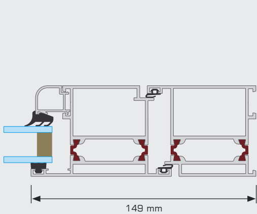
przekrój drzwi
