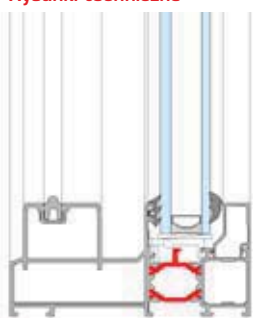
Ościeznica / skrzydło rozwiązanie jedno szynowe
