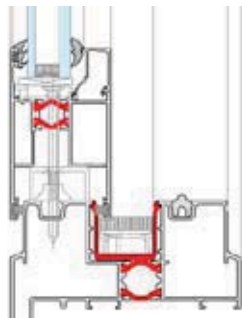
Kombinacje dwuszynowe Ościeznica / skrzydło z niewidocznym odwodnikiem
