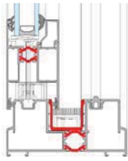
Ościeznica / skrzydło rozwiązanie dwuszynowe
